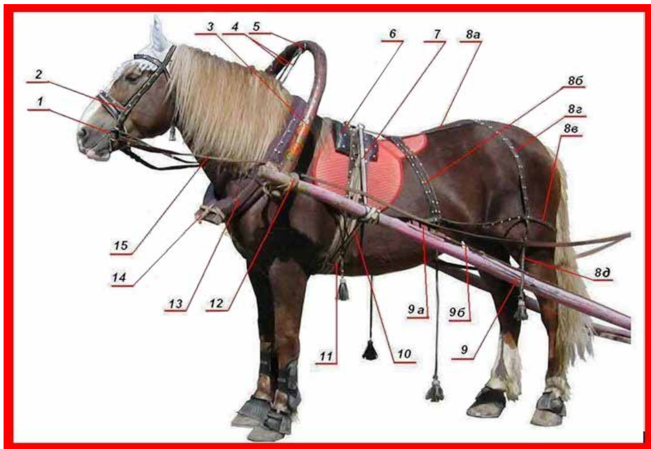
Сбруя для оглобльно-дуговой ("русской") запряжки. 1 - Удила; 2 - Узда; 3 - Дуга; 4 - Повод с темляком; 5 - Зга; 6 - Седелка; 7 - Чересседельник; 8 - Шлея : а) продольный ремень, б) поперечные ремни, в) откосный ремень, г) ободовый ремень, д) мочка; 9 - Оглобля: а) гребенка, б) тяж; 10 - Подбрюшник; 11 - Подпруга; 12 - Гуж; 13 - Хомут; 14 - Супонь; 15 - Вожжи
